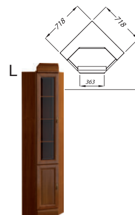
BA-14 regał narożny L, P** W: 2423 S: 273 G: 380
