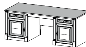
ME-2 biurko wolnostojące W: 760 S: 1920 G: 800
