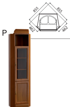
BA-13 regał barek** W: 2423 S: 462 G: 462
