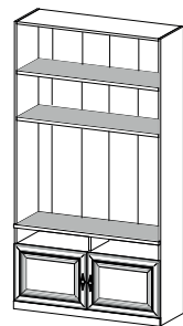
ME-9 panel RTV W: 2290 S: 1200 G: 410
